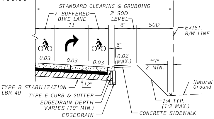
DETAIL LIMITS STA. 2190+85.00 - STA. 2191+15.00
