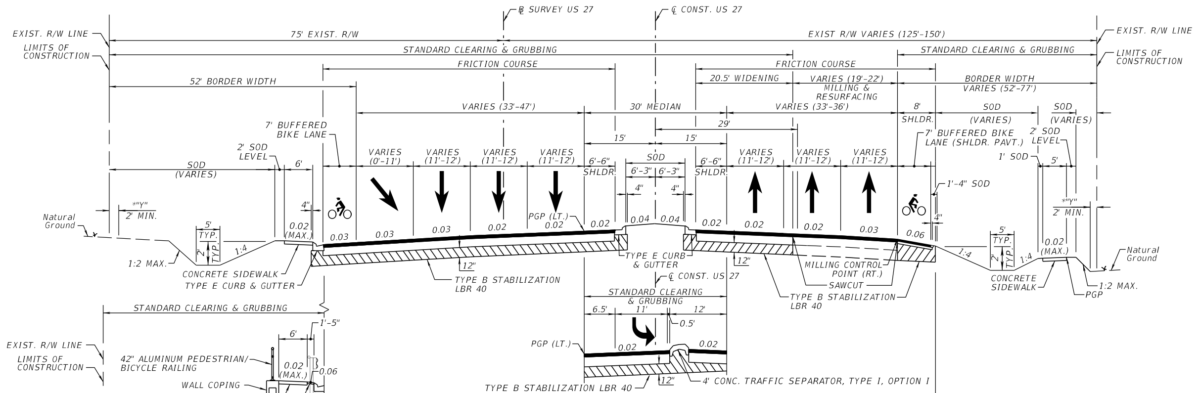
DETAIL LIMITS STA. 2179+50.00 - STA. 2183+10.00
